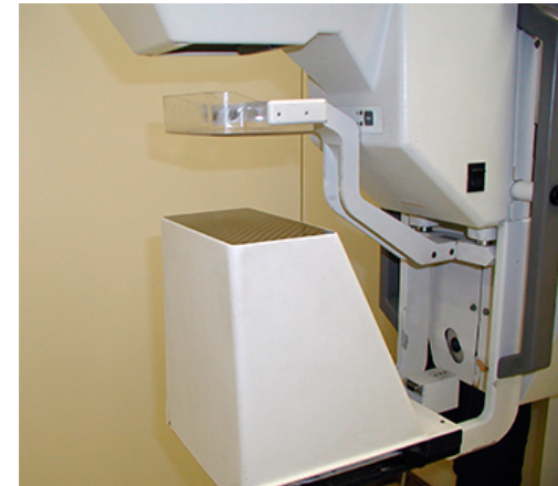
Figura 68. Manobra associação entre compressão seletiva e ampliação geométrica, acessórios (dispositivo de ampliação e compressor)
