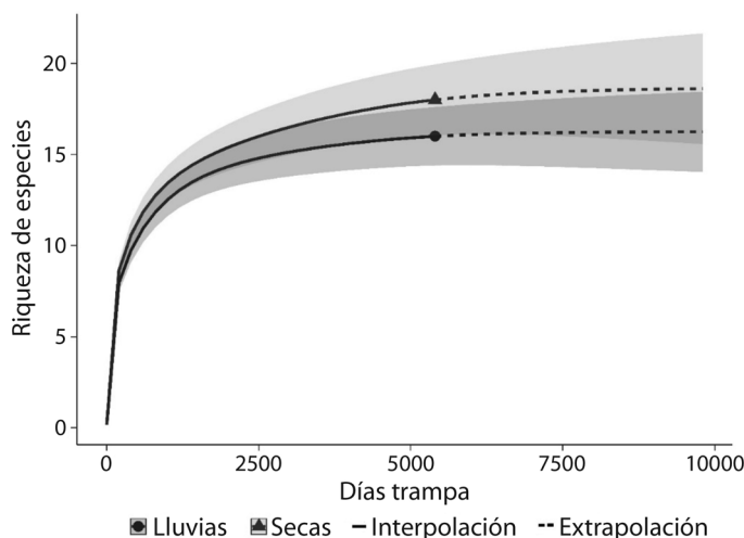
Fig. 1. Curvas de interpolación y extrapolación basadas en el esfuerzo de muestreo (días-trampa) para la riqueza de especies de mamíferos ( q = 0 ). Las muestras de referencia se señalan con símbolos (círculo: lluvias; triángulo: secas). La zona sombreada señala los intervalos de confianza al 95 %. La extrapolación se extiende hasta el doble del esfuerzo de muestreo de referencia.
