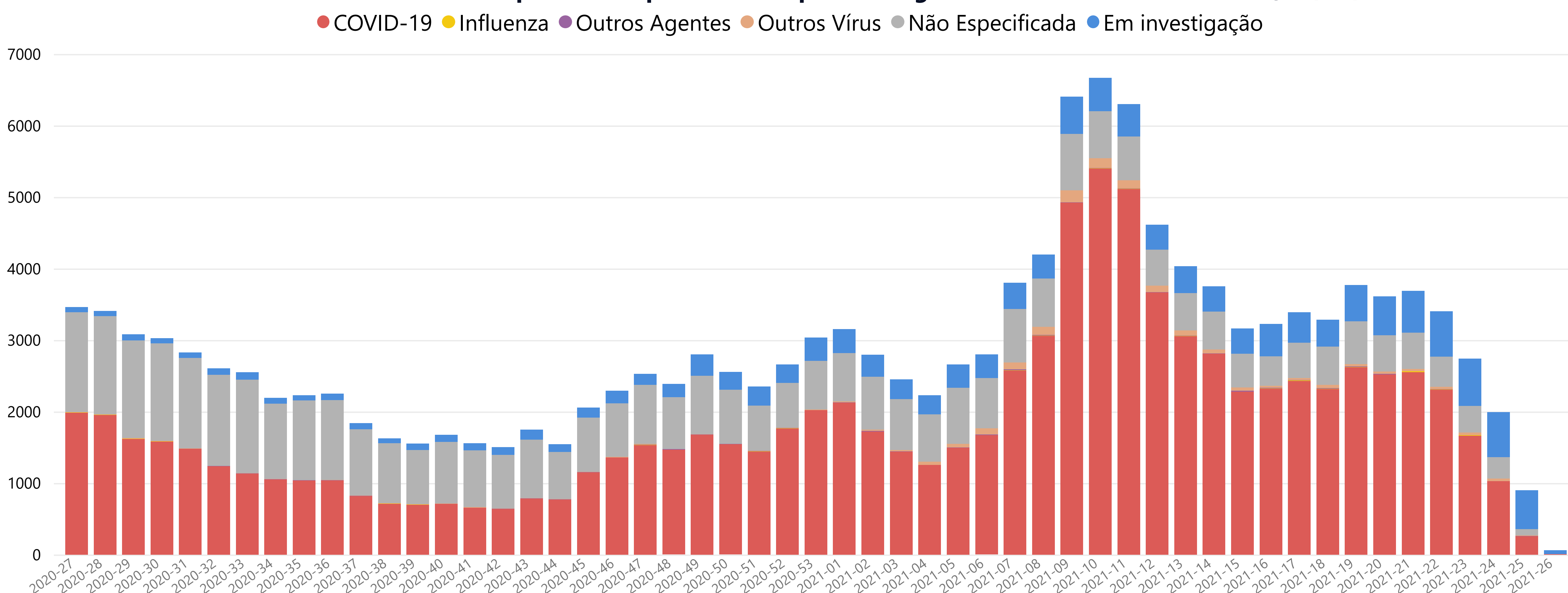
Casos notificados de SRAG hospitalizados por semana epidemiológica do início de sintomas. MSP, 30/06/2021
