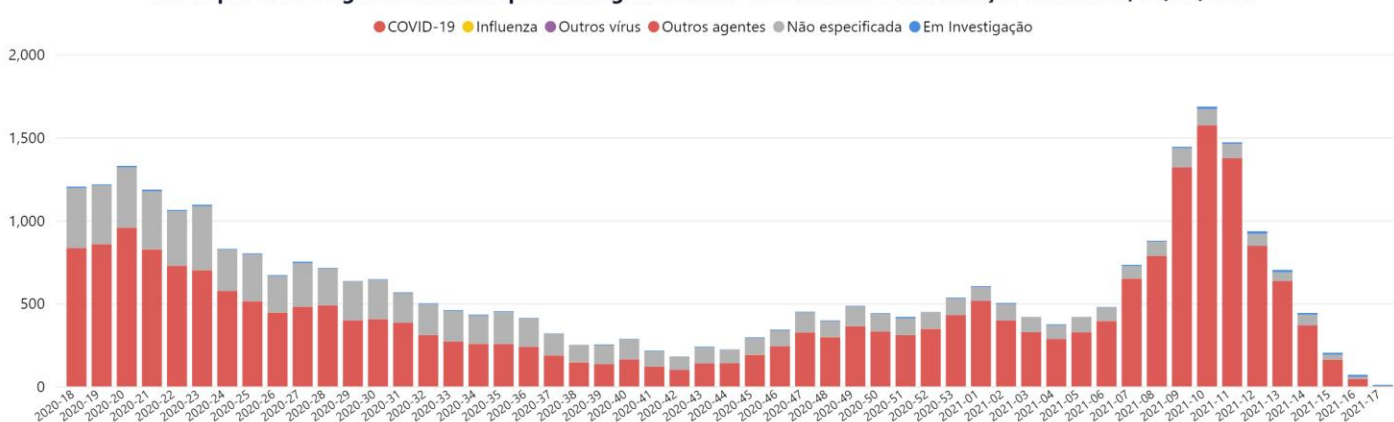
Óbitos por SRAG segundo semana epidemiológica de início de sintomas e classificação final. MSP, 01/05/2021
