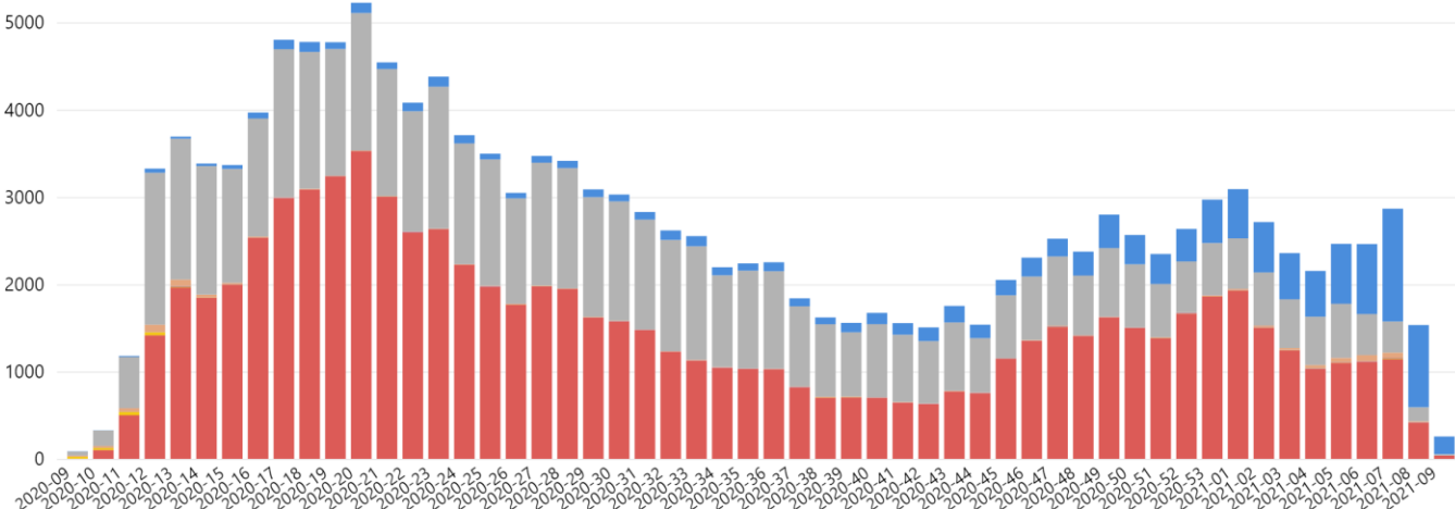
Casos notificados de SRAG hospitalizados por semana epidemiológica do início de sintomas. MSP, 04/03/2021
